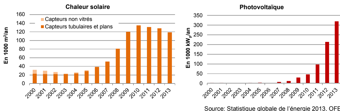
Figure 1 Evolution de la vente annuelle d'énergie solaire
